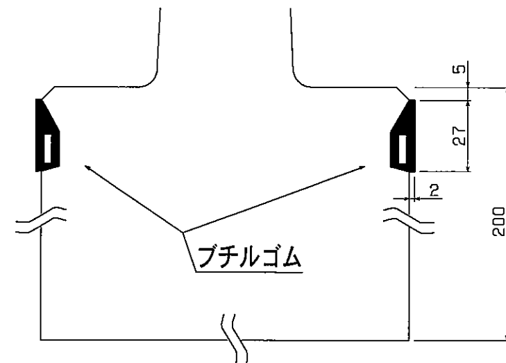
ブチルゴム設置図
