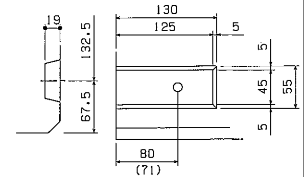
連結プレート詳細
